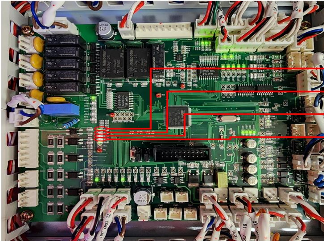
PCB1 Board / (JC-P13-V9.0)
